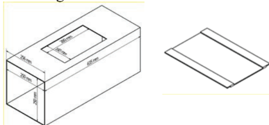
Hình 3.1 Buồng thử
