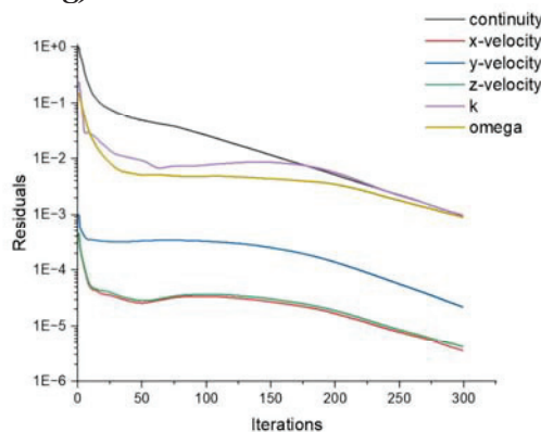
Hình 4.5 Biểu đồ kiểm tra độ hội tụ của mô phỏng số 2
